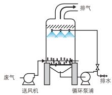
废气洗涤塔
